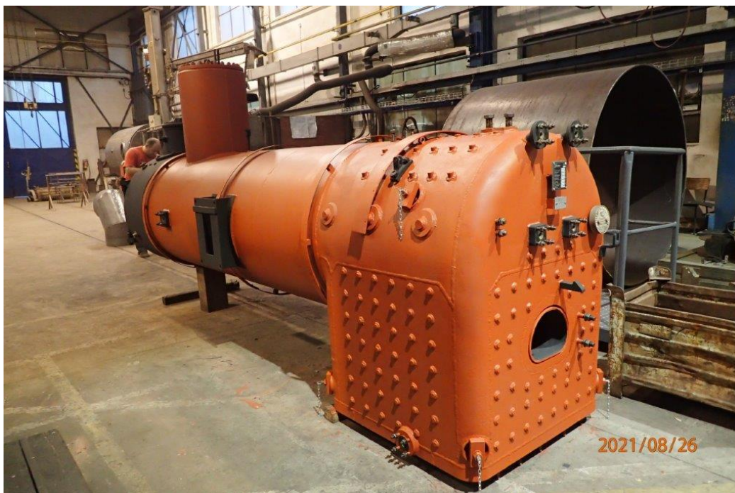
Parný kotol lokomotívy Katka
